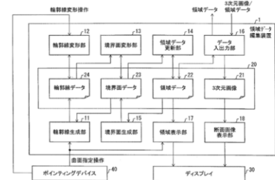
領域データ編集装置のブロック図
